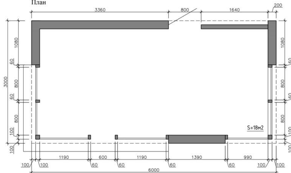
План
