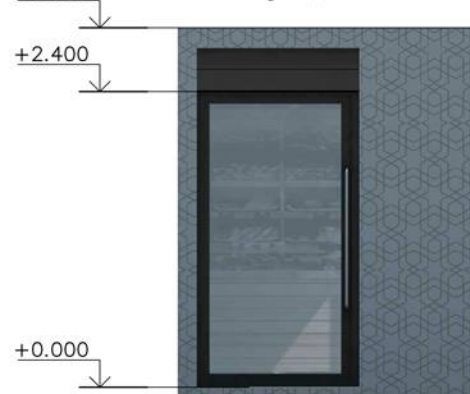
Боковой фасад
