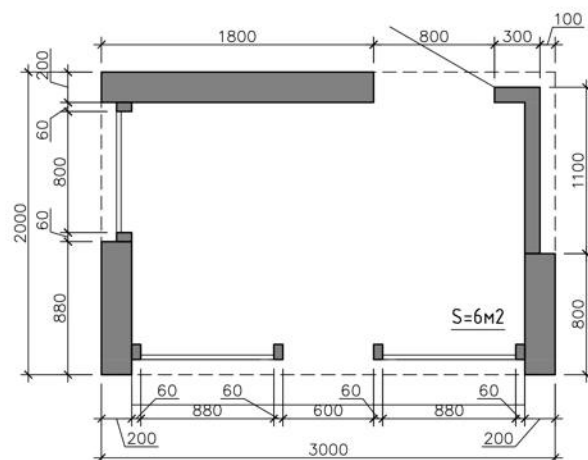
План
