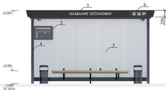
Лицевой фасад
