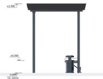
Боковой фасад
